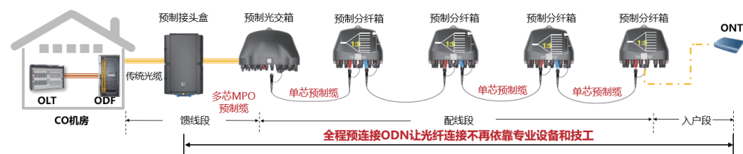
图 4-1 预连接 ODN 典型路由图
