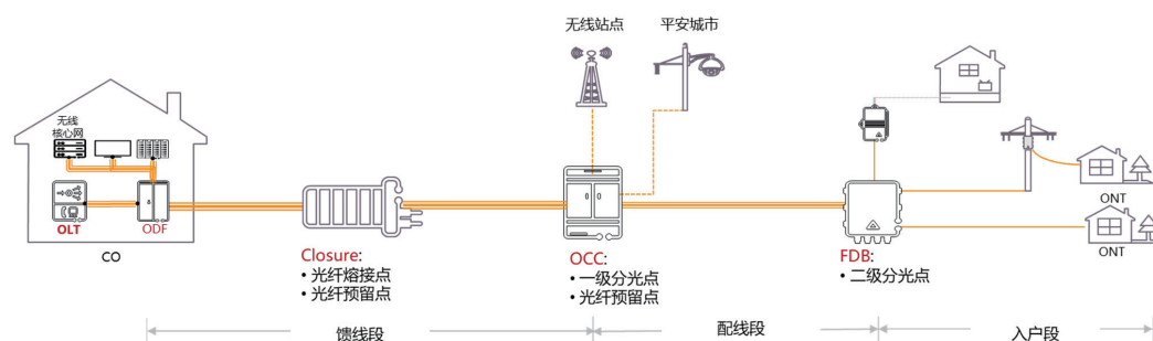
! 图 2-1 ODN 网络结构示意图 !
