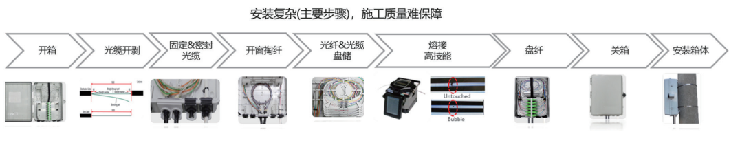
❗ 图 3-1 光纤连接步骤 ❗
