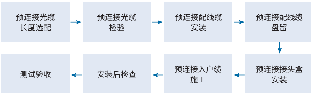
图 5-10 预连接 ODN 方案施工流程图
