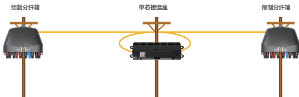
❗ 图 5-6 光缆段延长接续示意图 ❗
