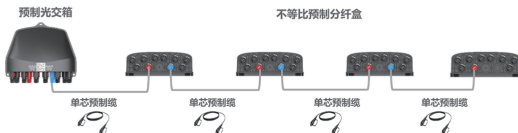
图 4-4 基于预连接技术的不等比组网示意图
